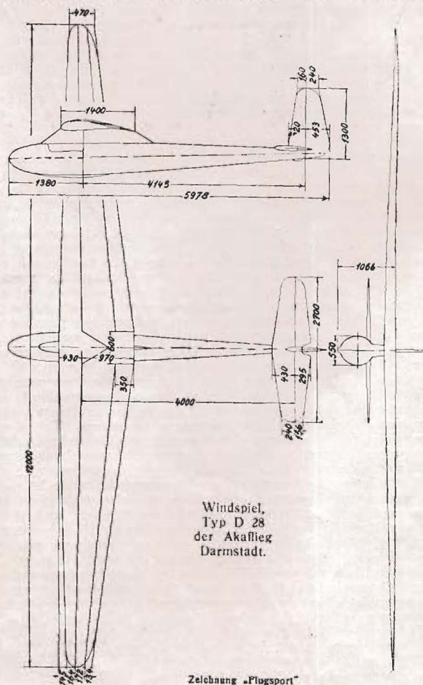
Zeichnung „Flugsport“
